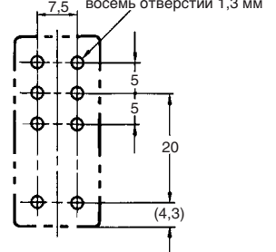
Крепежные отверстия
