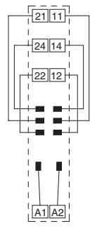
Расположение клемм (вид сверху)
